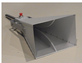
【ホーンアンテナ】 ・Schwarzbeck製 BBHA9120LF
