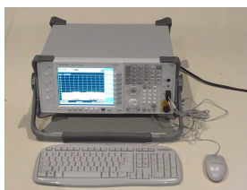
【スペクトラムアナライザ】 ・Agilent Technologies製 N9020A
