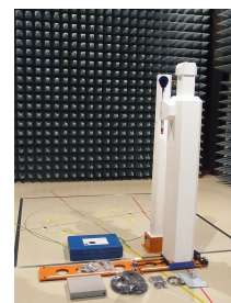
【SVSWR測定キット】 ・コロナ電子工業製 CSVS-001他 ・Seibersdorf製 MA4POD16
