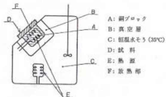
保温性試験機
