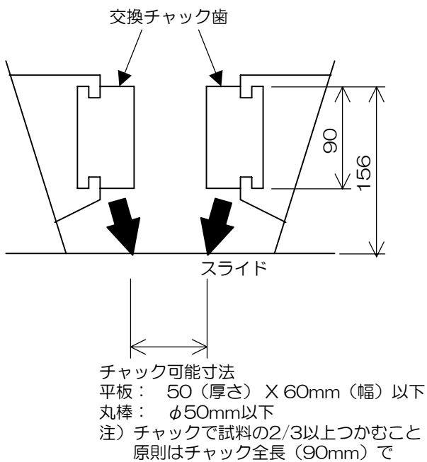
図3 引張試験片取付け部概寸
