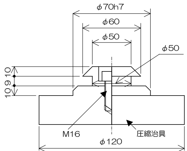
図4 圧子取付け部寸法
