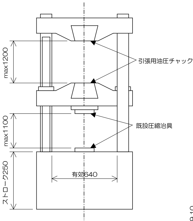
図1 試験機概寸
