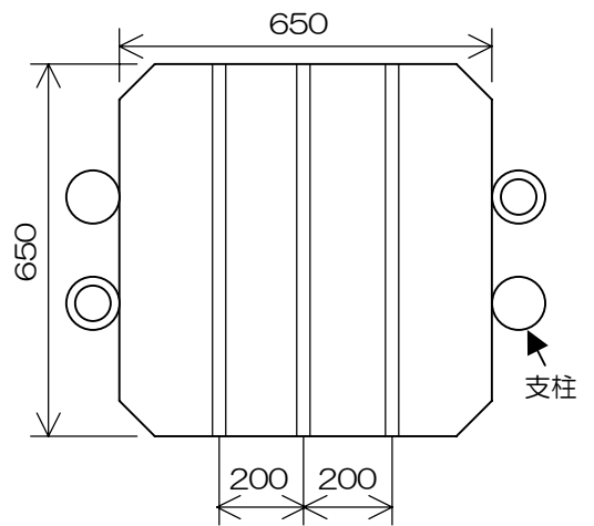
図2 ステージ寸法
