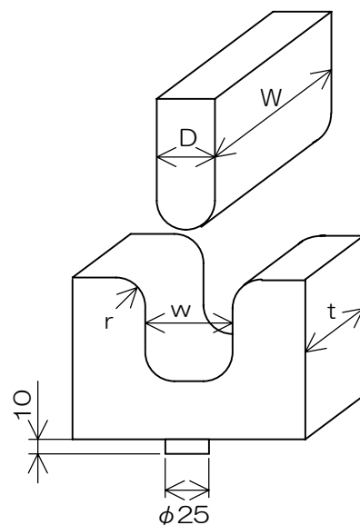
図5 型曲げ試験治具 (表1, 2参照)
